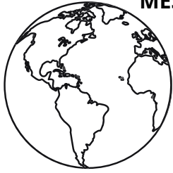
ZEMĚ
