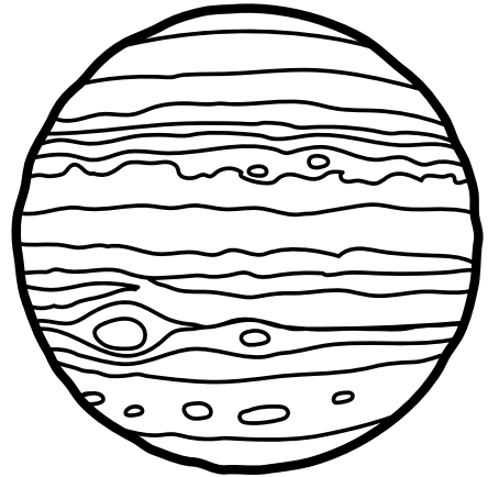
JUPITER
