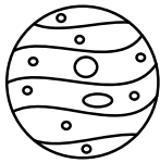
MERKUR
